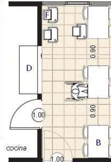
EJEMPLO 2 | 31.5m 2 - 36 plazas
