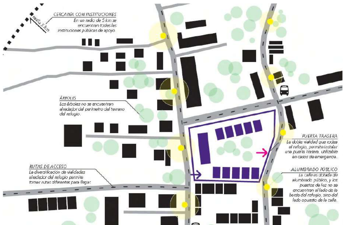
Imagen 15. Esquema de ubicación positiva (CONAVIM & ONU-HABITAT, 2016, pág. 25)
