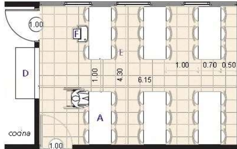
EJEMPLO 1 | 26.5m 2 - 36 plazas
